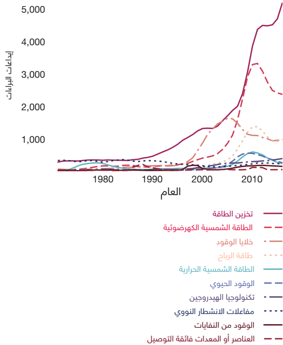
الشكل 3-3 ب تكنولوجيات تخفيف آثار تغير المناخ في مجال الطاقة حسب الفئات الفرعية
